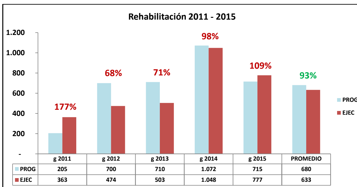
Gráfico Nº 5 Kilómetros en Rehabilitación 2011 - 2015
