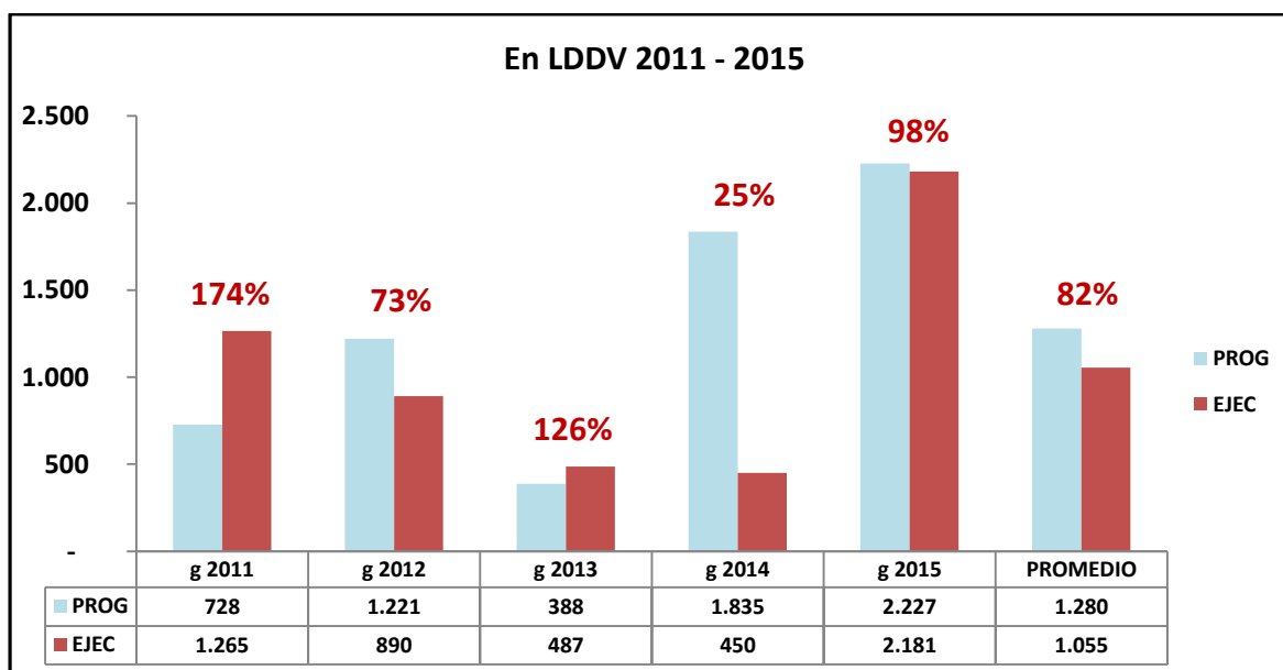
Gráfico Nº 6 Kilómetros en Liberación del Derecho de Vía 2011 – 2015
