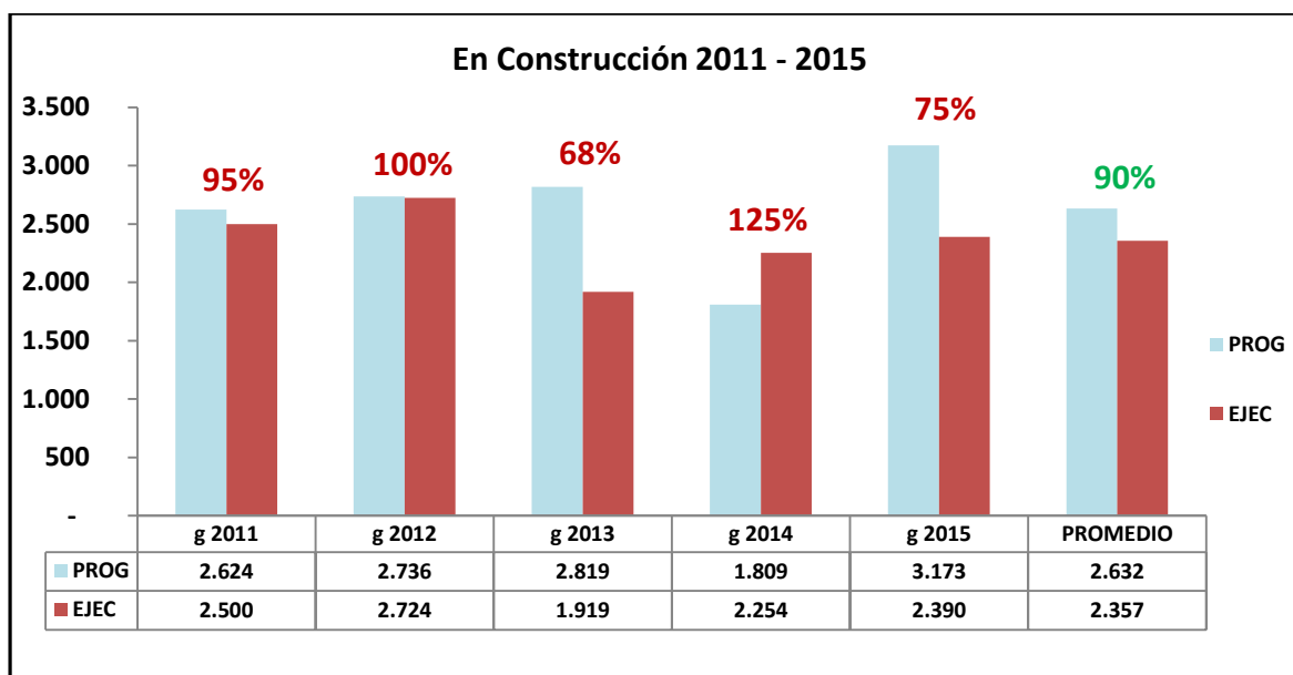
Gráfico N° 2 Kilómetros en Construcción 2011 - 2015
